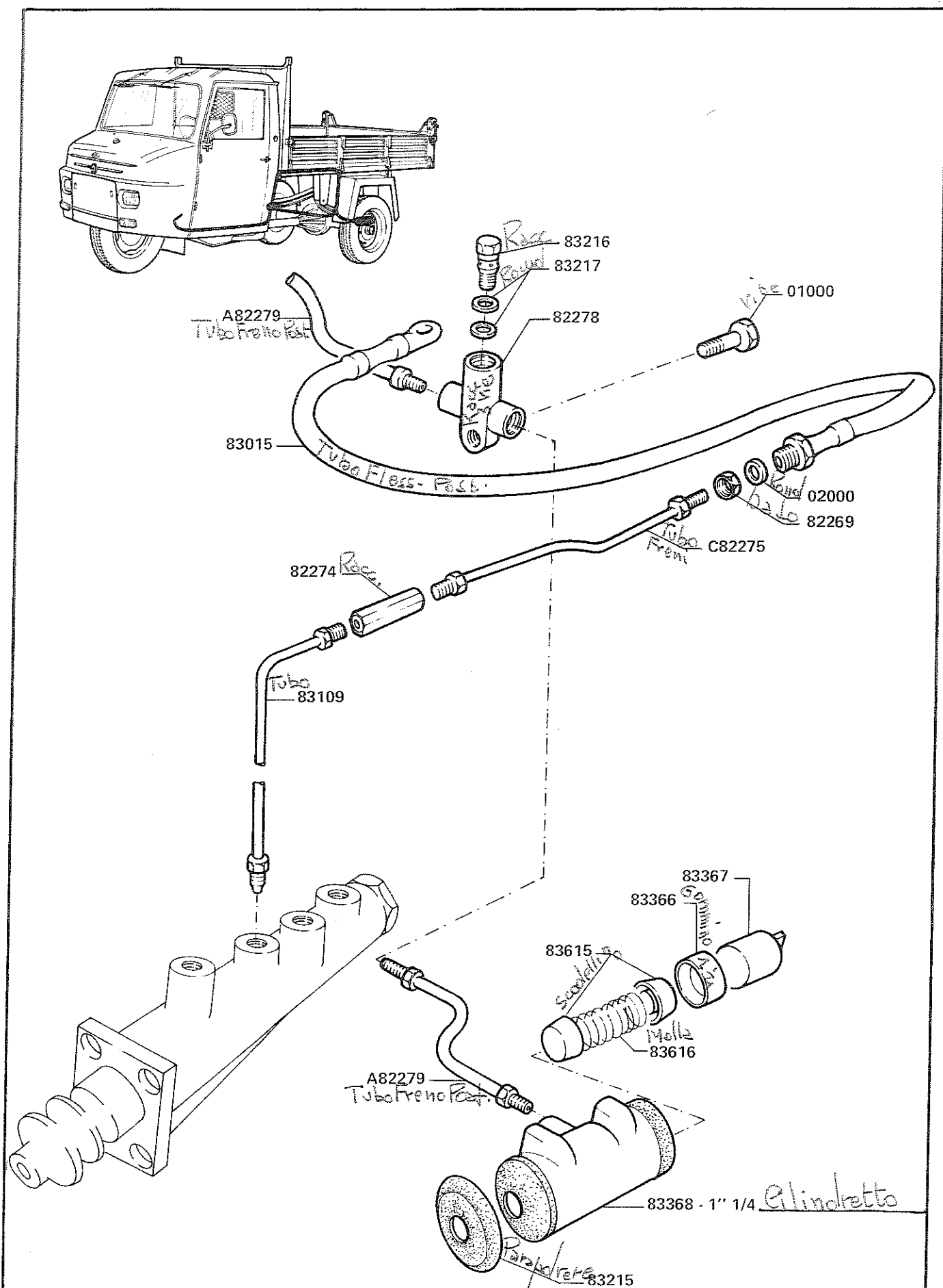
TAV. 26 - TUBAZIONE FRENO IDRAULICO POSTERIORE
