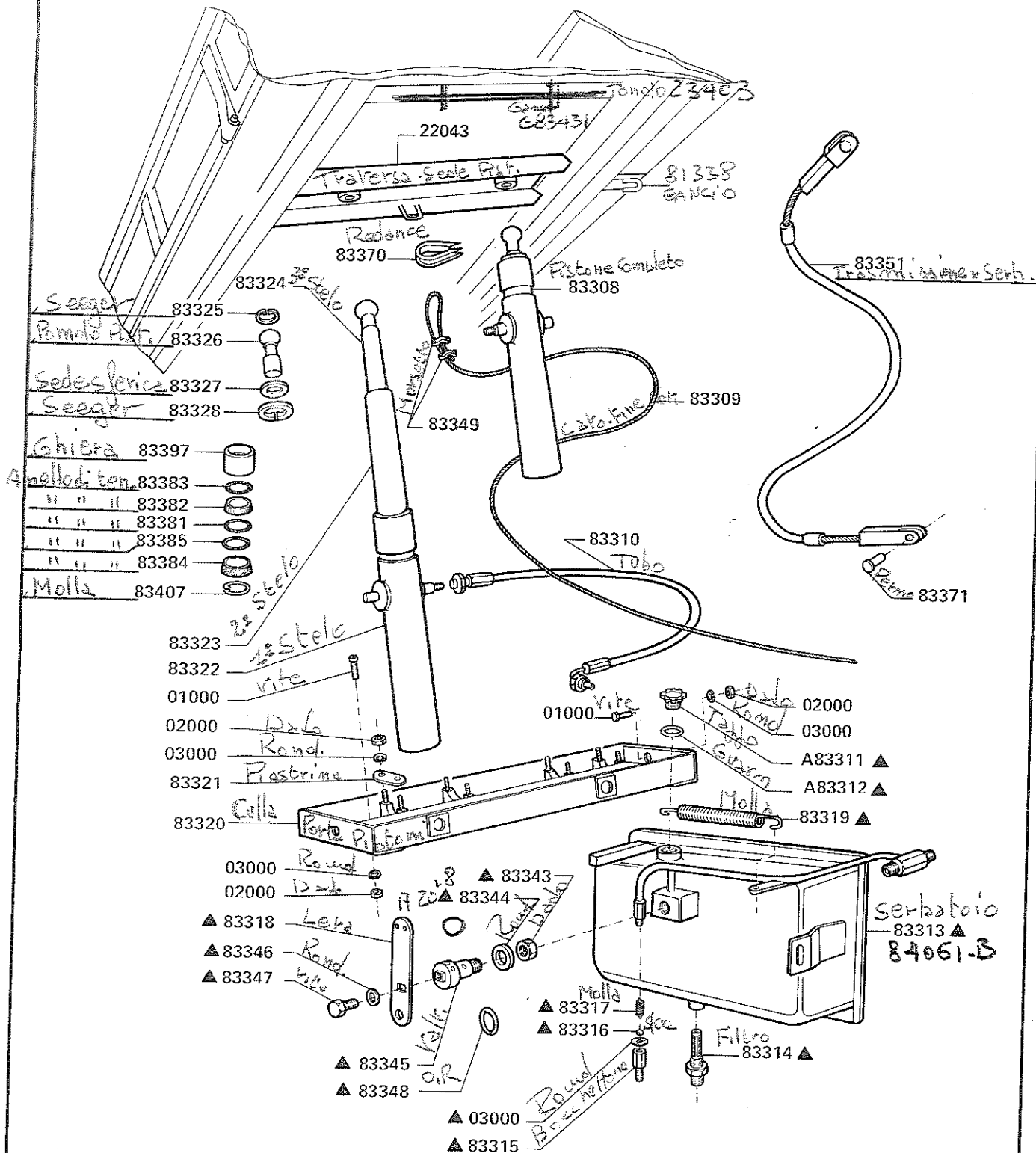
TAV. 36 – PISTONI CULLA E SERBATOIO
