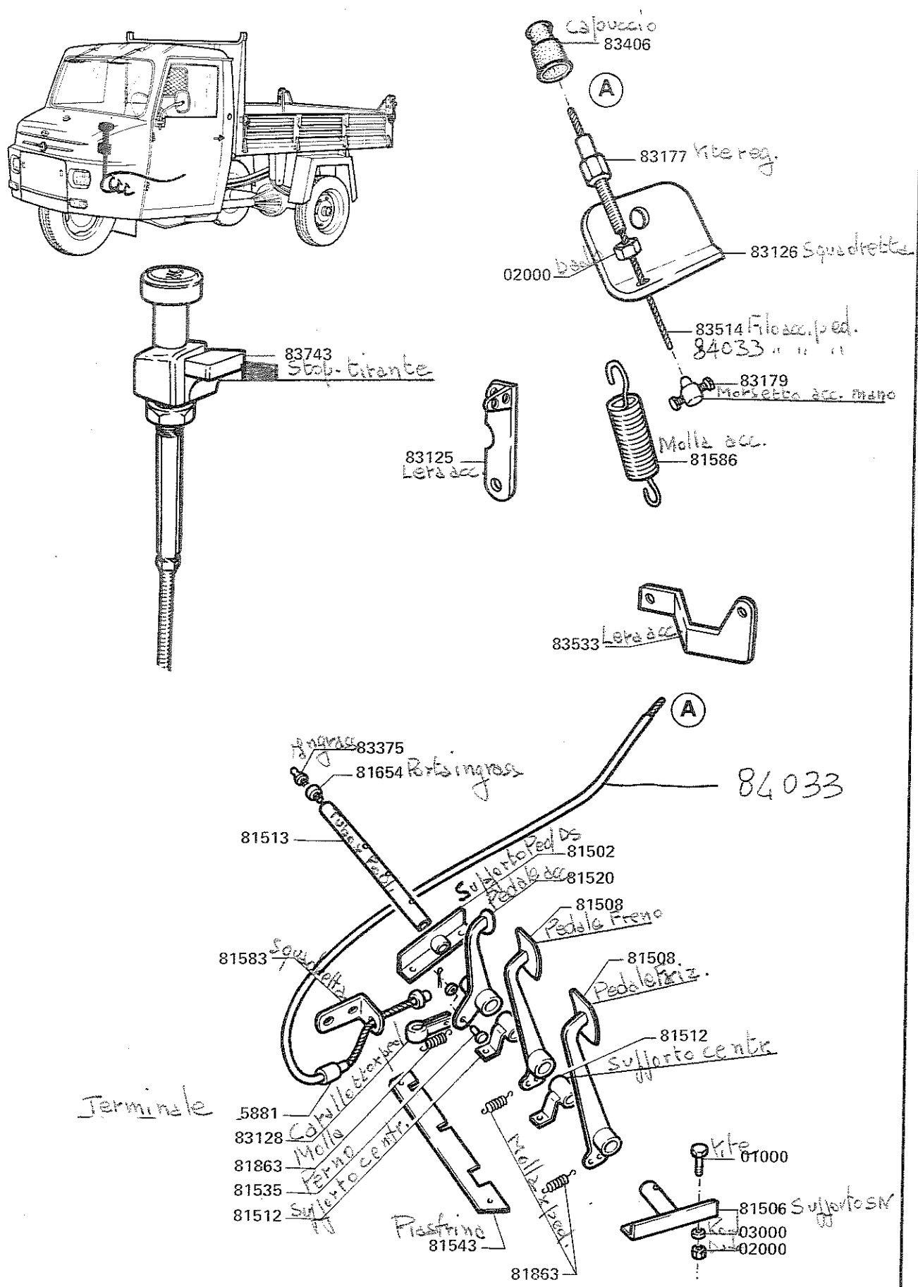
TAV. 24 - PEDALIERA E COMANDI - FIG. 1/2
