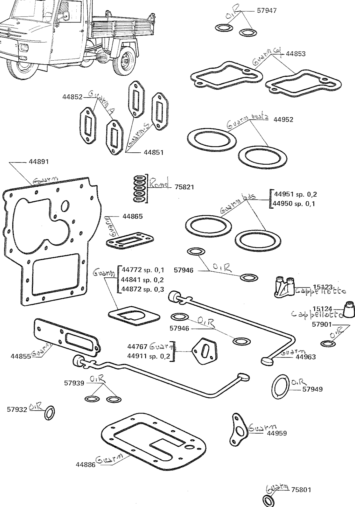
TAV. 45 – GUARNIZIONI PER RD 952
